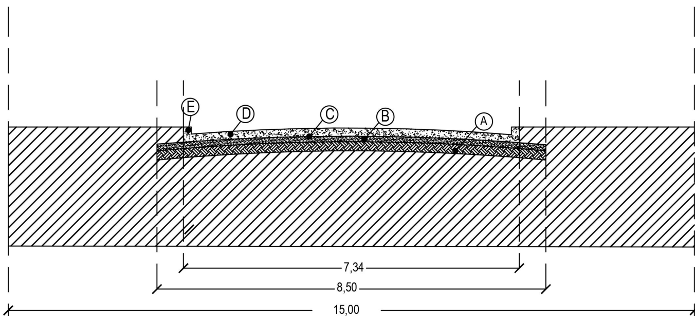
CORTE TRANSVERSAL
